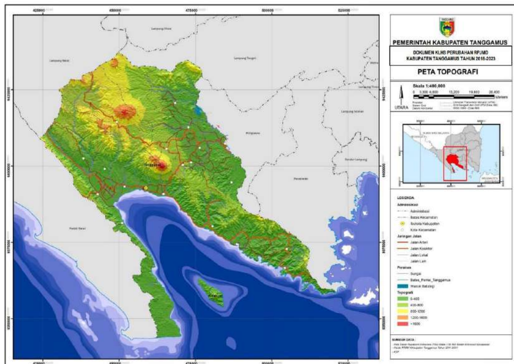
Gambar II.5. Peta Topografi Kabupaten Tanggamus
