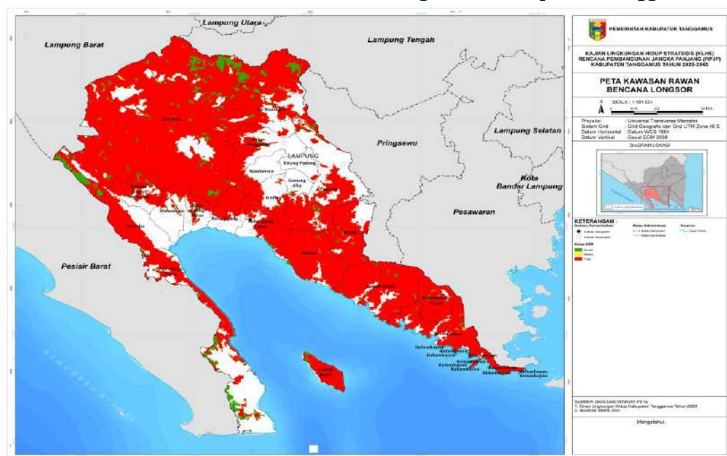
Gambar II.10. Peta Kerentanan Tanah Longsor di Kabupaten Tanggamus
