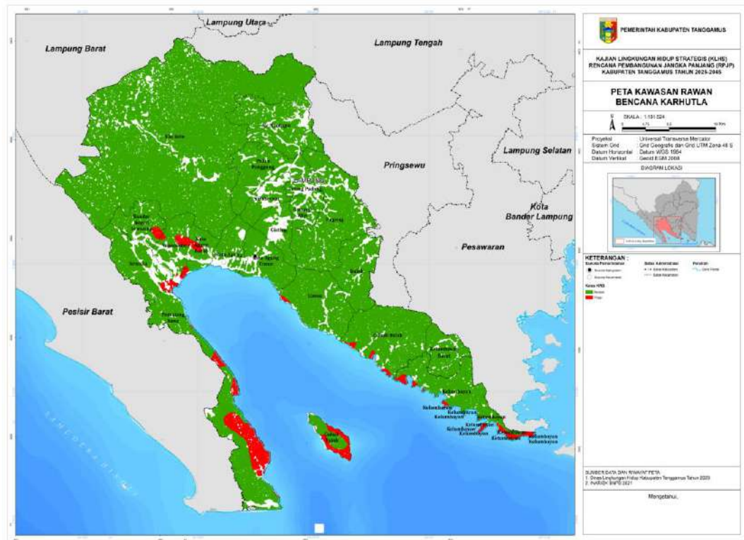
Gambar II.14. Peta Kerentanan Kebakaran Lahan dan Hutan di Kabupaten Tanggamus
