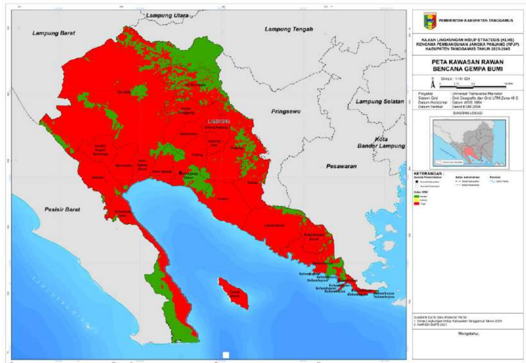
Gambar II.12. Peta Kerentanan Gerakan Tanah di Kabupaten Tanggamus
