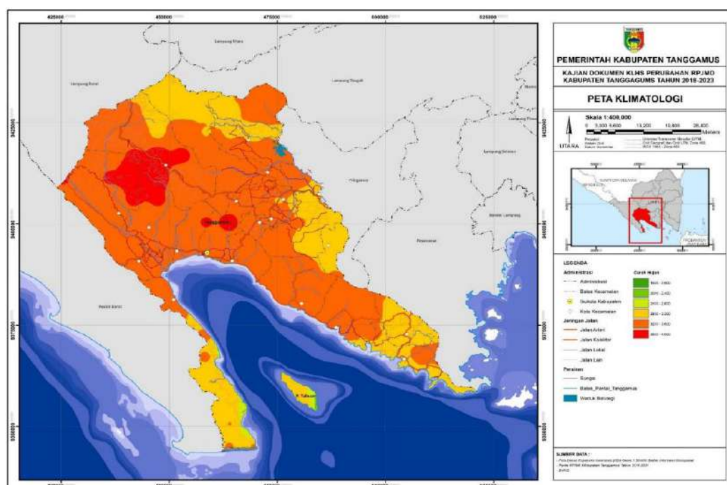
Gambar II.8. Peta Klimatologi Kabupaten Tanggamus
